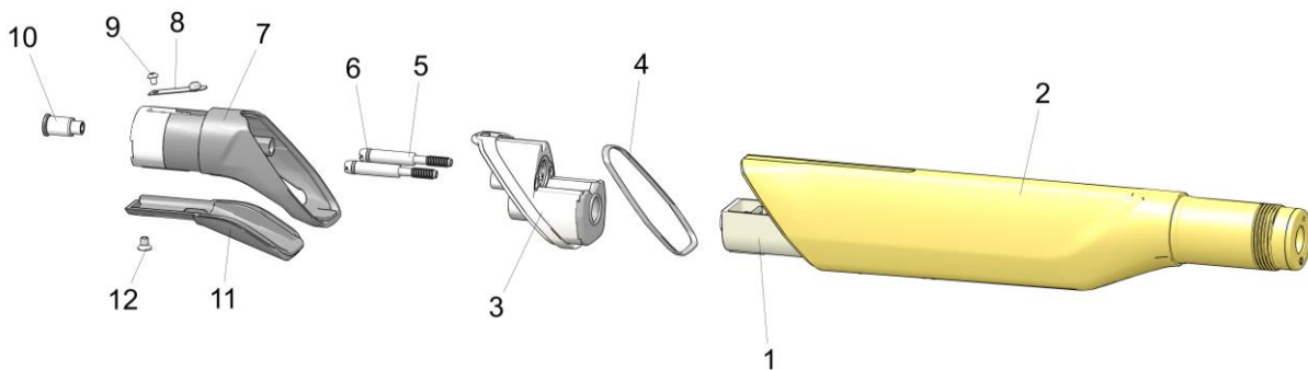
fig. 12: OptiGun GA03 – shaft
